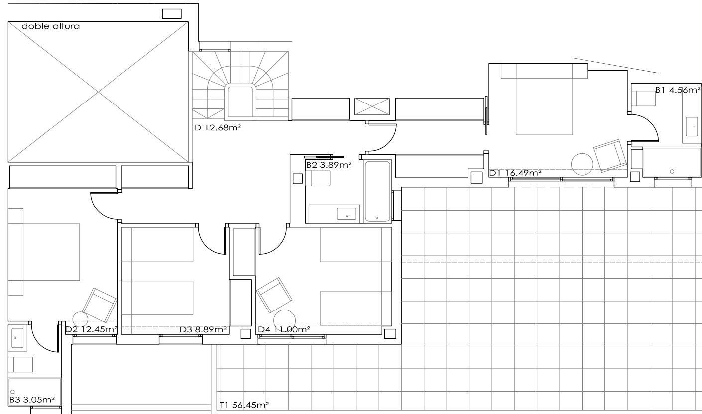
Planta superior
