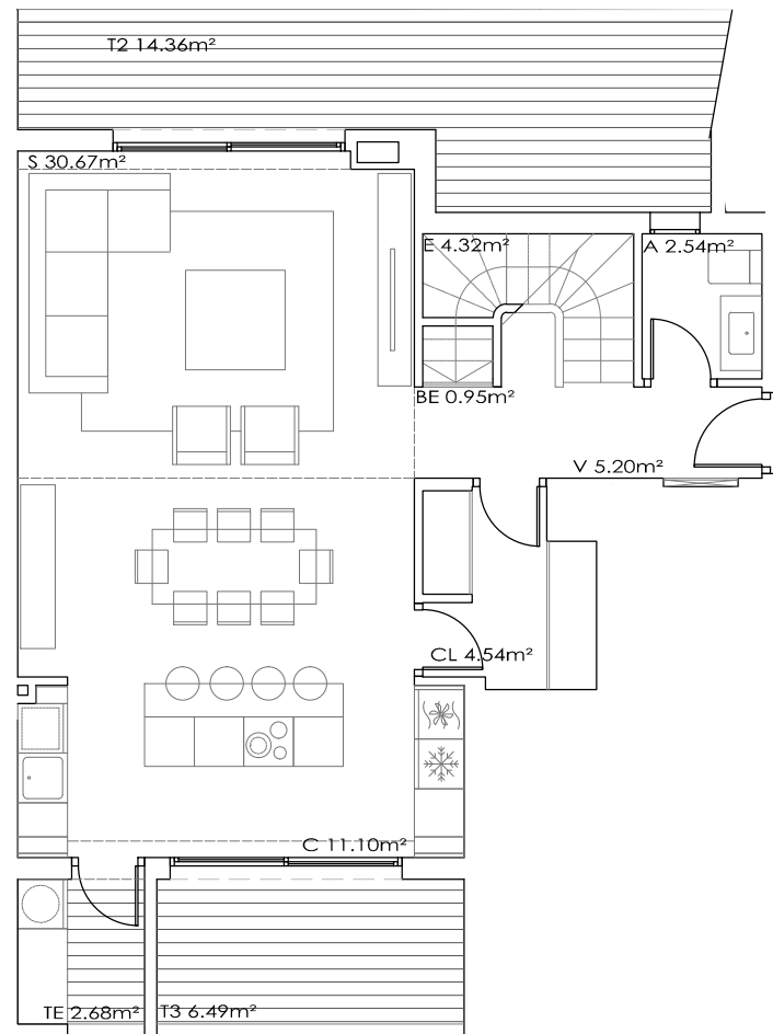
Planta inferior
