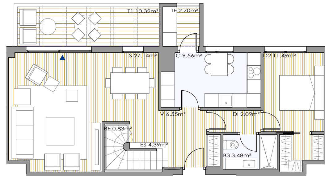
Planta inferior
